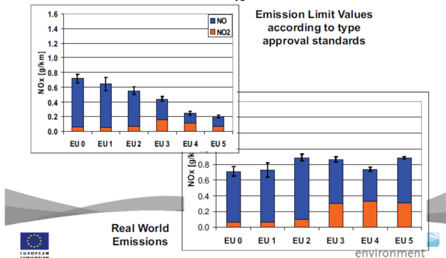
Figuur 2: Evolutie van de NOx- en NO 2 emissie van dieselpersonenvoertuigen volgens de testcyclus (links) en in werkelijkheid (rechts). Bron: presentatie van S. Hausberger (TU Graz) op NO 2 -workshop, 14-15 april 2010, Brussel.
